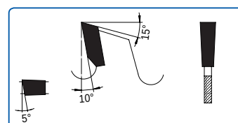
Abb.: Flachzahn mit Achswinkel (F, AW)
