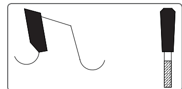
Abb.: Trapez Zahn (T)
