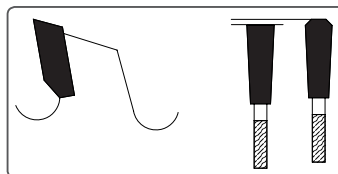
Abb.: Flach-Trapezzahn (FT)
