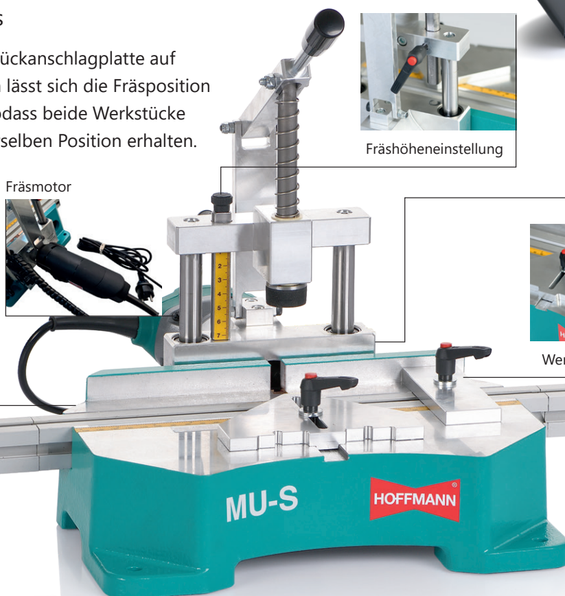
Fräshöheneinstellung
